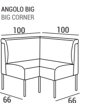
ANGOLO BIG BIG CORNER 100 100 66 66
