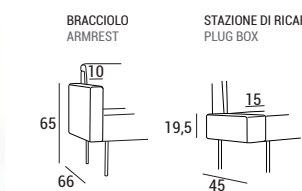
BRACCIOLO ARMREST STAZIONE DI RICARICA PLUG BOX
