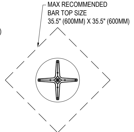
BAR PLAN
