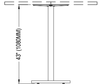
BAR ELEVATION
